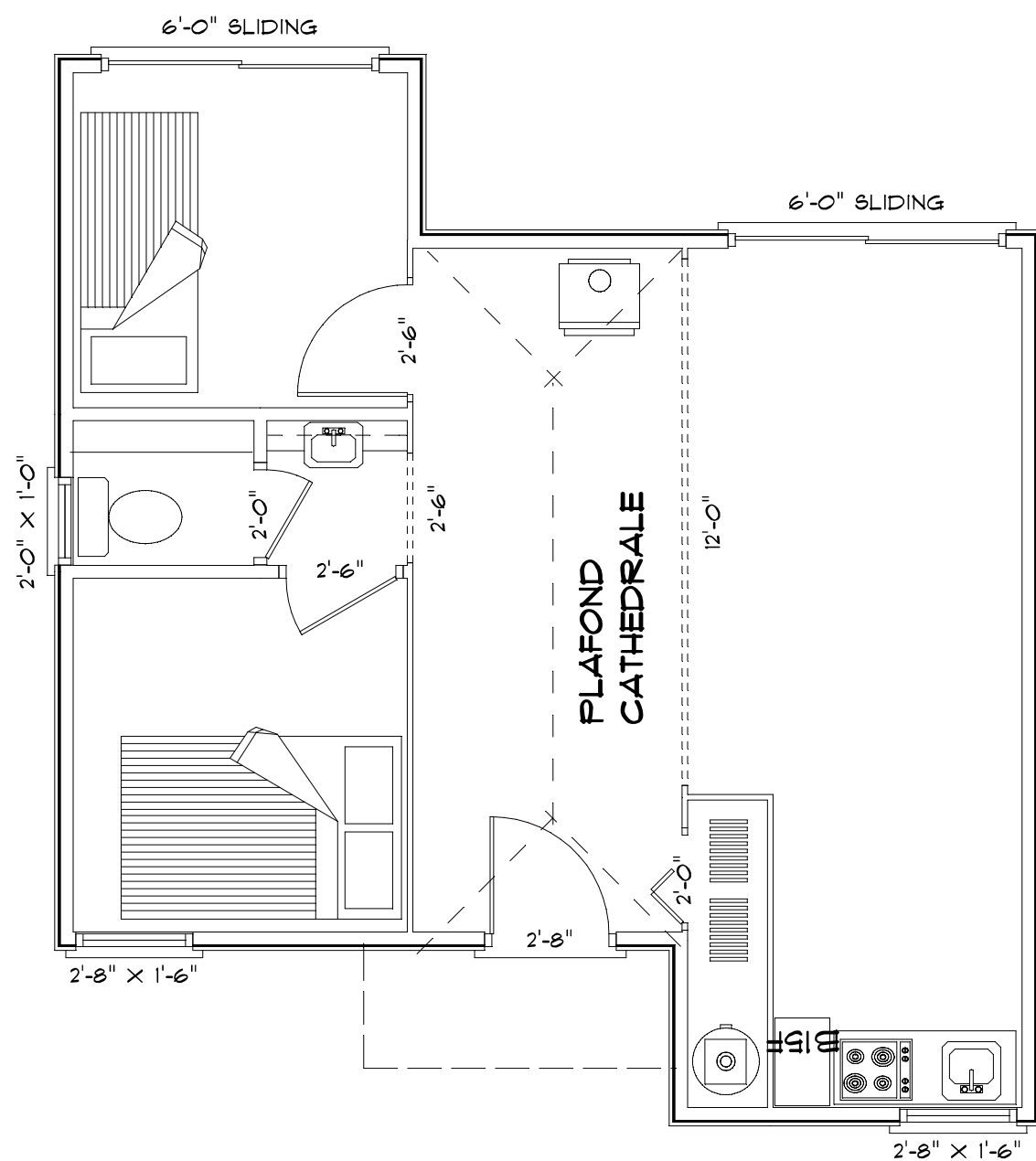
PLAN E PAVILLON 460 P.C.
