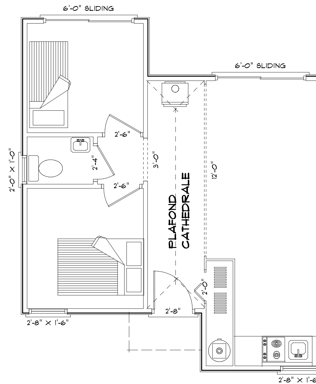
PLAN F PAVILLON 421 P.C.
